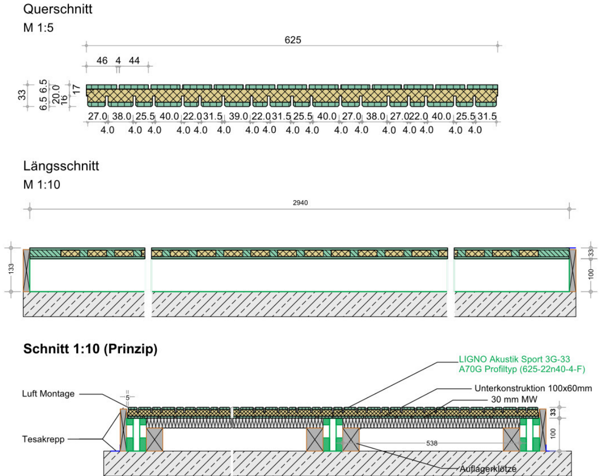
Bild 5: Prüfaufbau (Herstellerangabe)
