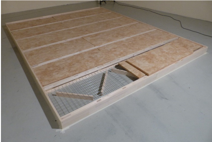
Bild 1: Rahmenkonstruktion mit Bedämpfung
