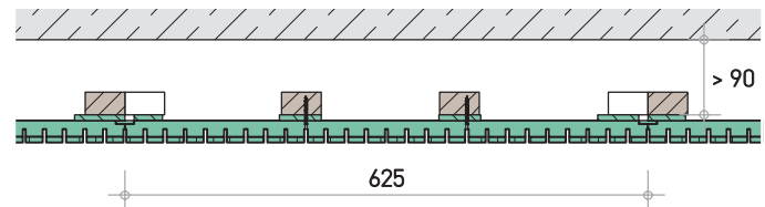
Querschnitt
