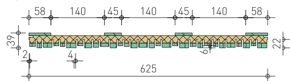
Querschnitt:
