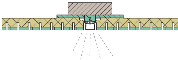
Montage flächenbündig:
