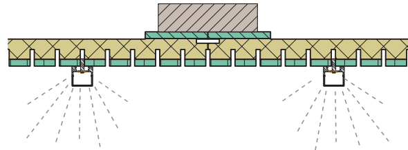
Aufsteckmontage:
