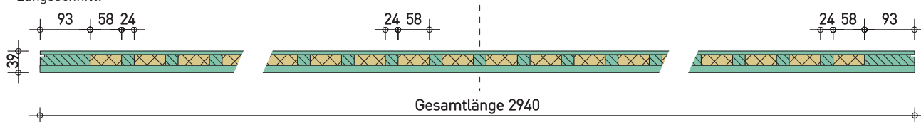
Längsschnitt:
