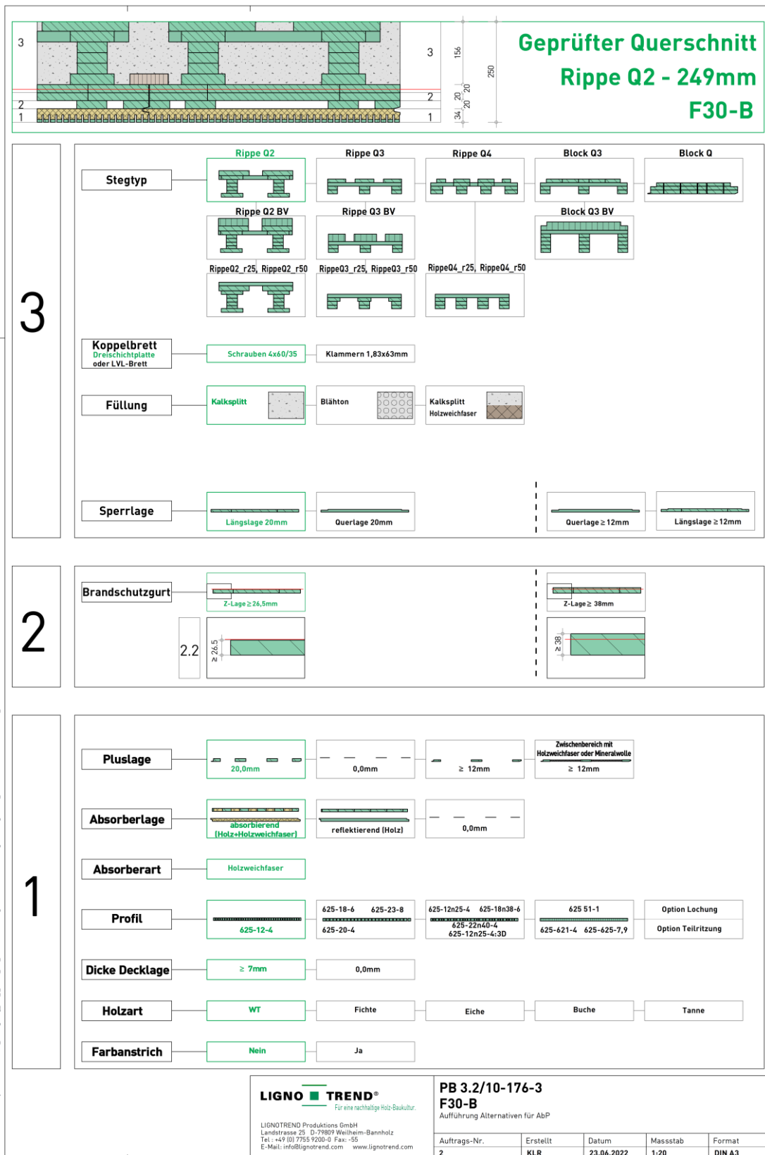
Abbildung A1.1 Skizzierter Aufbau der Lignotrend Deckenelemente der Feuerwiderstandsklasse F30-B unterteilt nach den einzelnen Aufbauebenen
