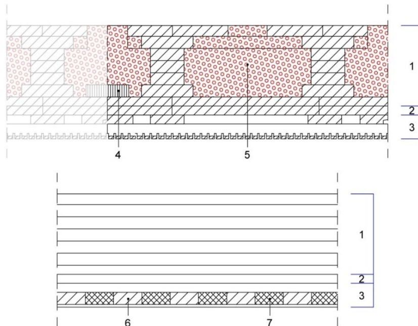
Abbildung 1: Beispielkonstruktion als Prinzipskizze – allgemeiner Aufbau eines Lignotrend - Deckenelementes
